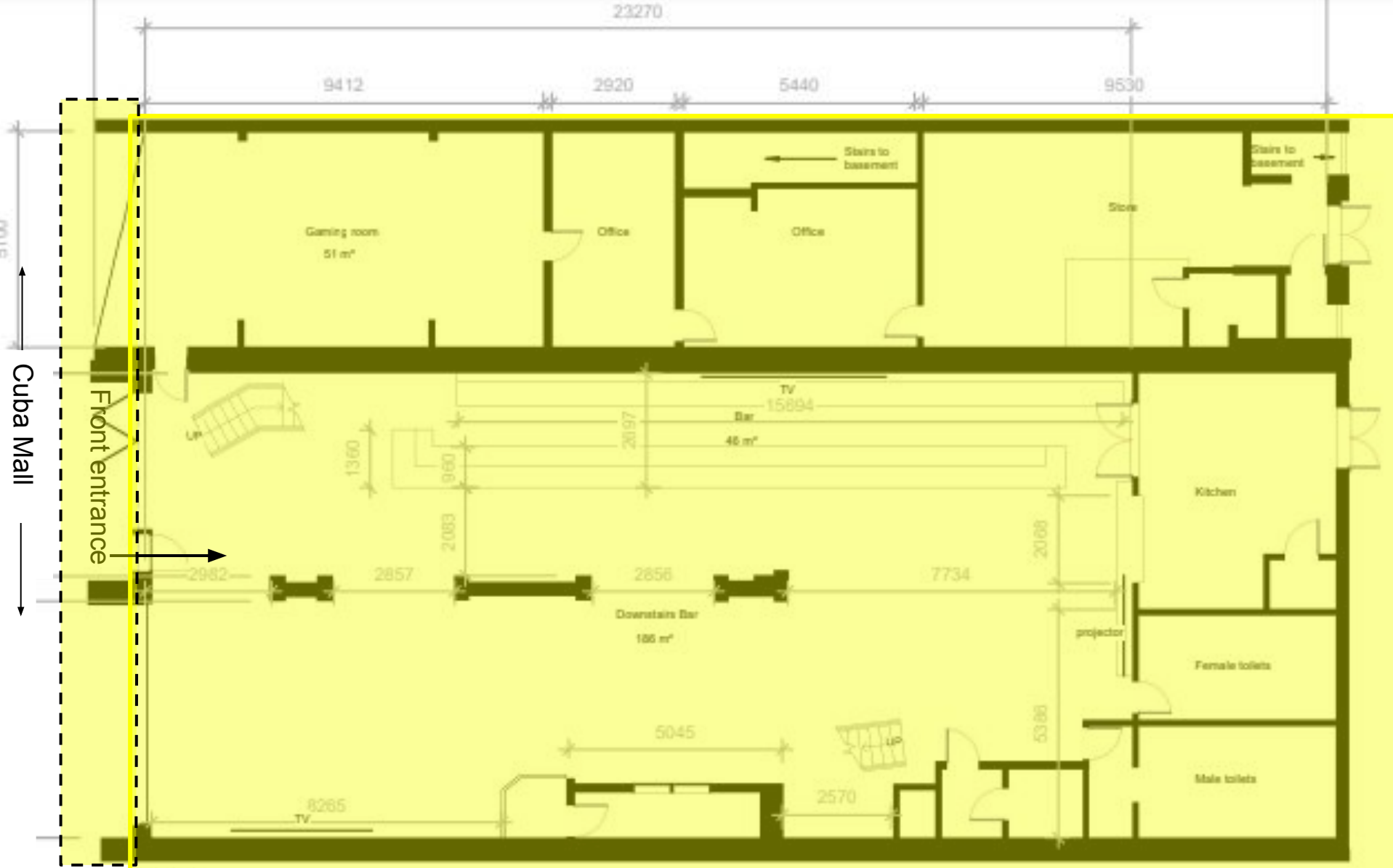
1 Level 1 1 : 100
