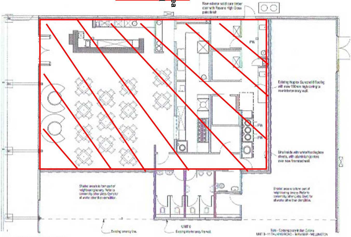
CARPENTRY SETOUT PLAN 1:100 Scale
